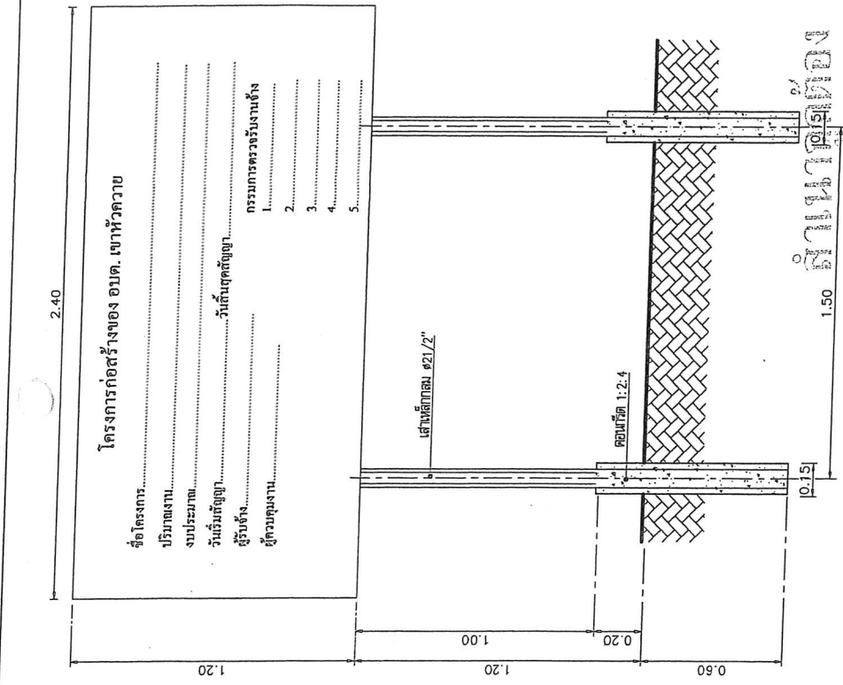
แบบมาตรฐานป้ายประธาัมพันธ์ อบต. มาตราส่วน 1:20
